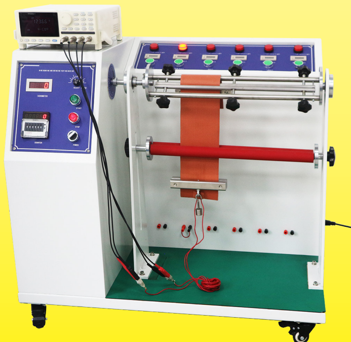
Гибкий силиконовый нагреватель при проведении испытания на сгибание
